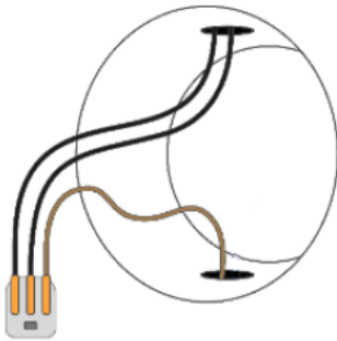
Abb. 9: Schließen Sie den Versorgungsstrom an der Anschlussklemme von Schalter 1 an
