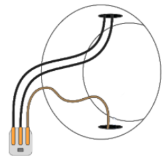
Fig. 6: Branchez l'alimentation à la borne de connexion
