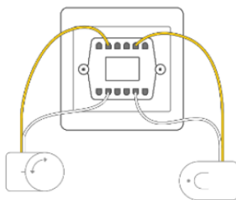
Fig. 7: Connectez le convertisseur d'interrupteur à l'interrupteur d'éclairage
